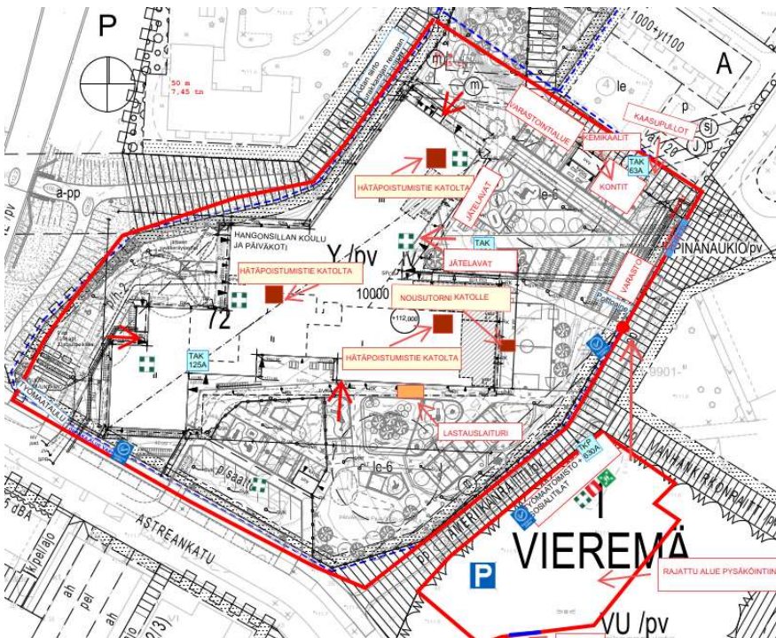
Työmaasuunnitelma.
