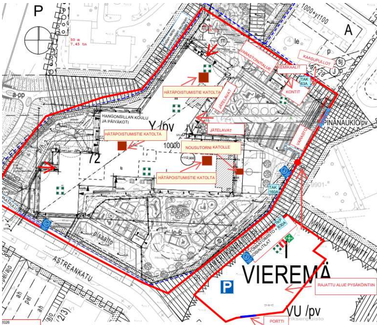
Työmaasuunnitelma.
